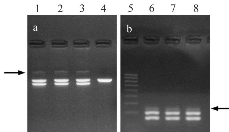
Рис. 3.10 Утворення гетеродуплексів при ампліфікації гетерозиготних зразків.
